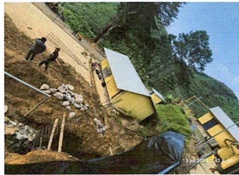
Foto 2: Avance de muro de contención, así mismo Zanjeo
